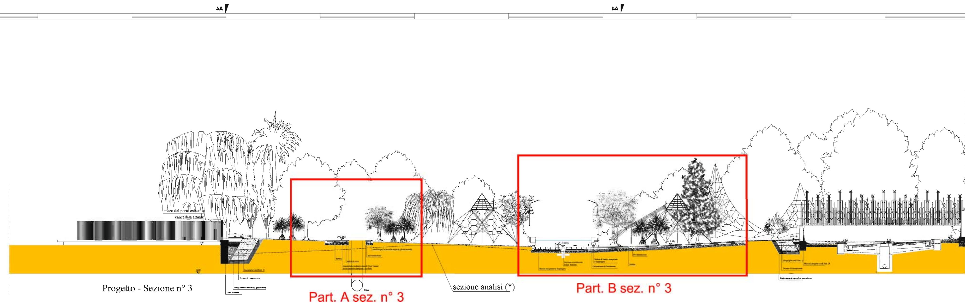
Sezione di progetto n° 3 - scala 1:200
