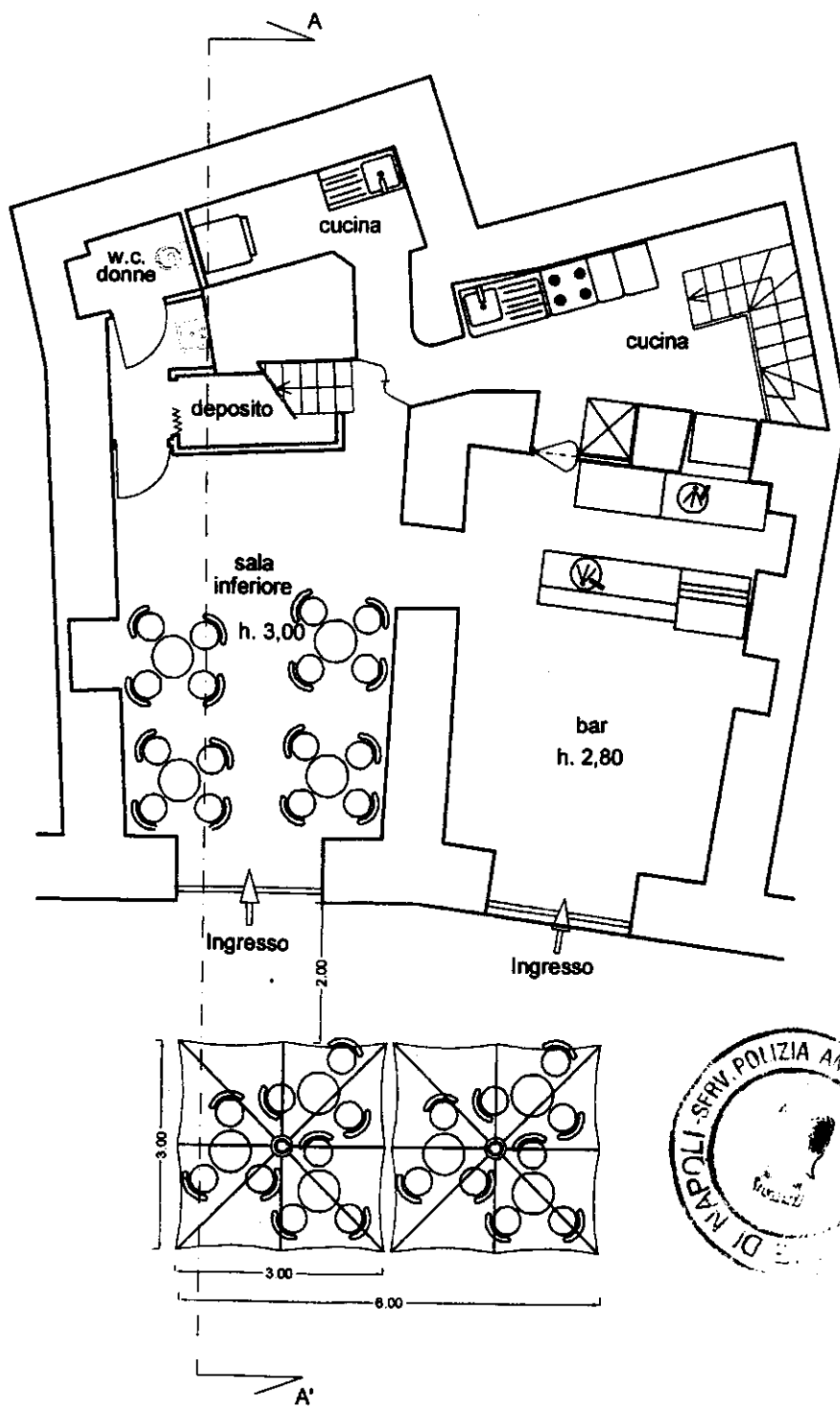
Planimetria scala 1:100
