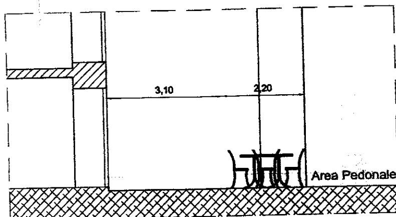
SEZIONE Stato di progetto Scala 1:100
