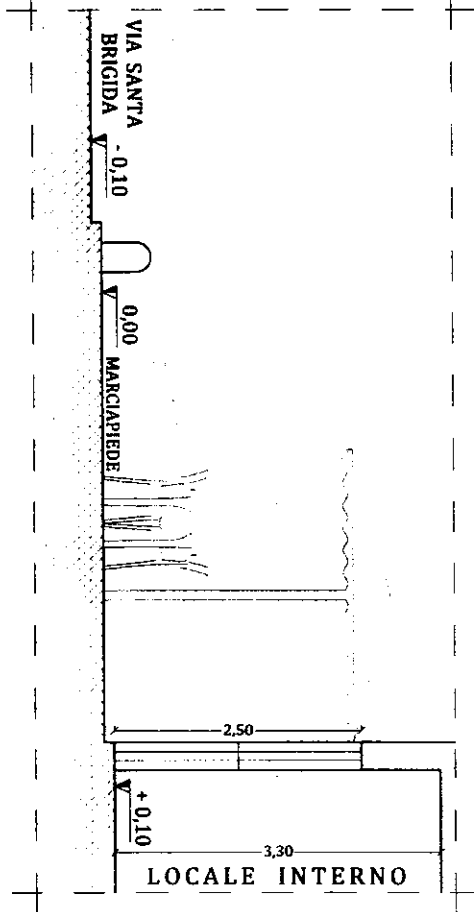
SEZIONE B - B' STATO DI PROGETTO - RAPP. 1:50
