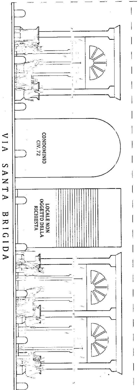
PROSPETTO LATO NORD STATO DI PROGETTO - RAPP. 1:50
