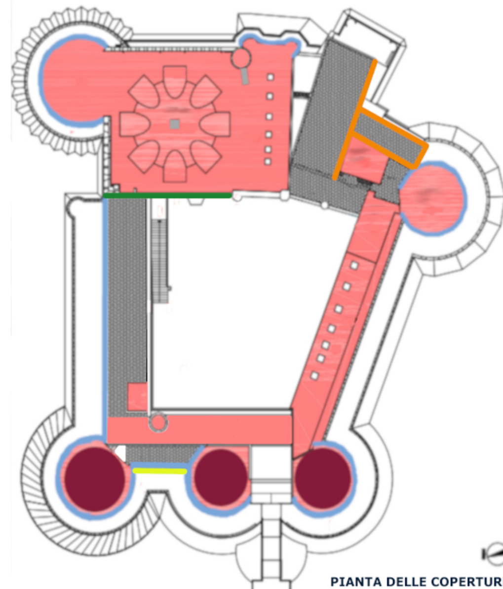
INTERVENTO N°06 INTERVENTO SULLA MURATURA ESTERNA IN TUFO SOTTOSTANTE LA LOGGIA TRA TORRE SAN GIORGIO E TORRE DI MEZZO
