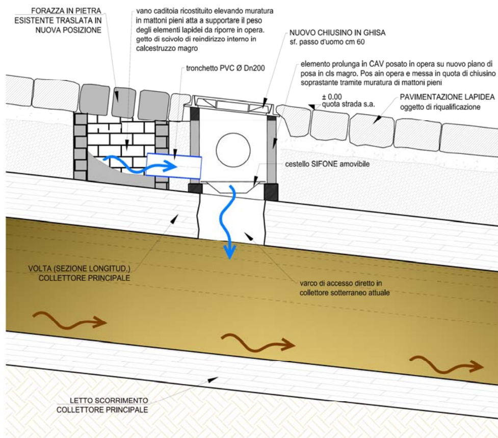
Figura 8 - soluzione spostamento caditoia storica a fessura e suo sifonamento
