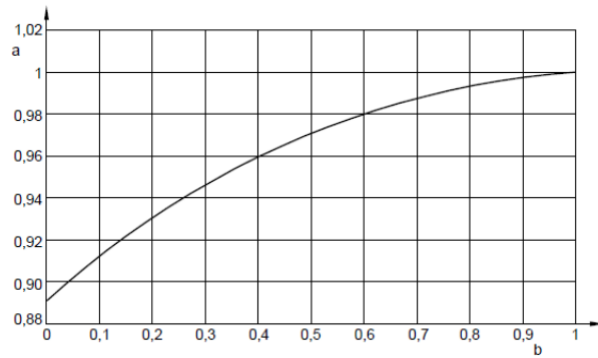
6 Coefficiente di forma, F_s Legenda a Coefficiente di forma F_s b S/T
