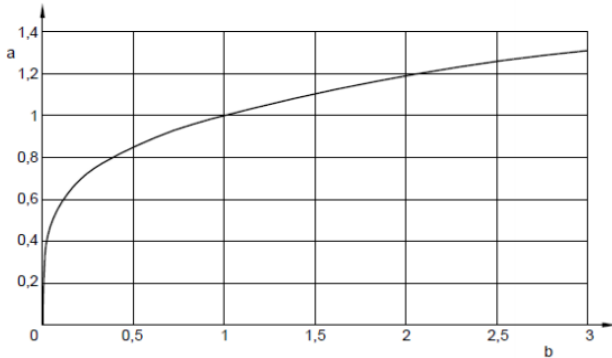
5 Coefficiente di altezza, F_d Legenda a Coefficiente di altezza F_d b W/T
