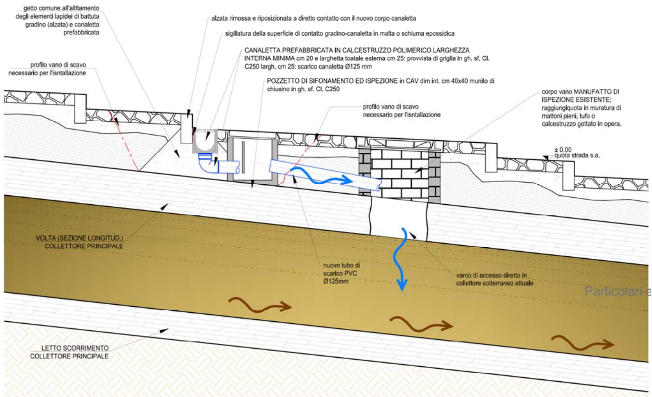
Figura 9 - inserimento di canalette a ridosso delle alzate gradinate esistenti
