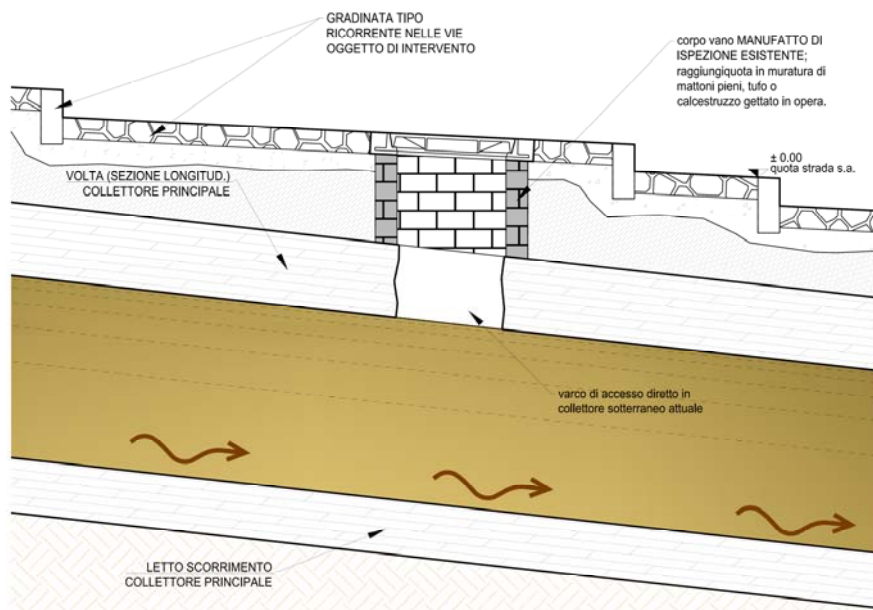
Figura 7 - torrino di ispezione tipo
