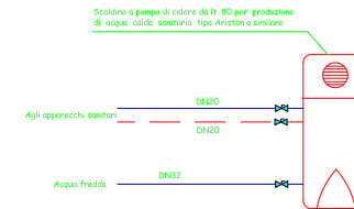
Schema di Impianto con scaldino a pompa di calore
