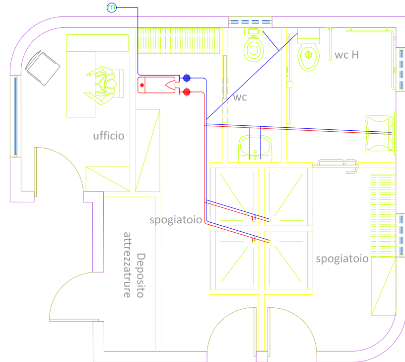
Schema di Impianto con scaldino a pompa di calore
