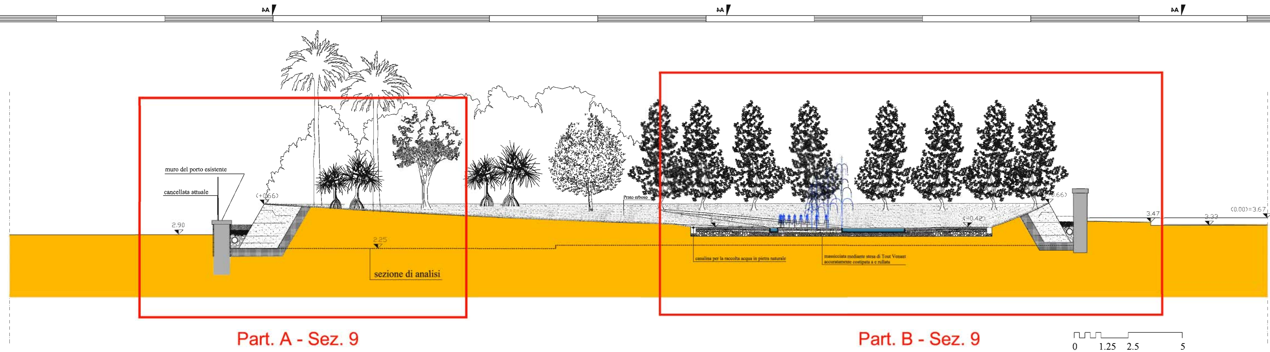
Sezione n° 9 di progetto - scala 1:100
